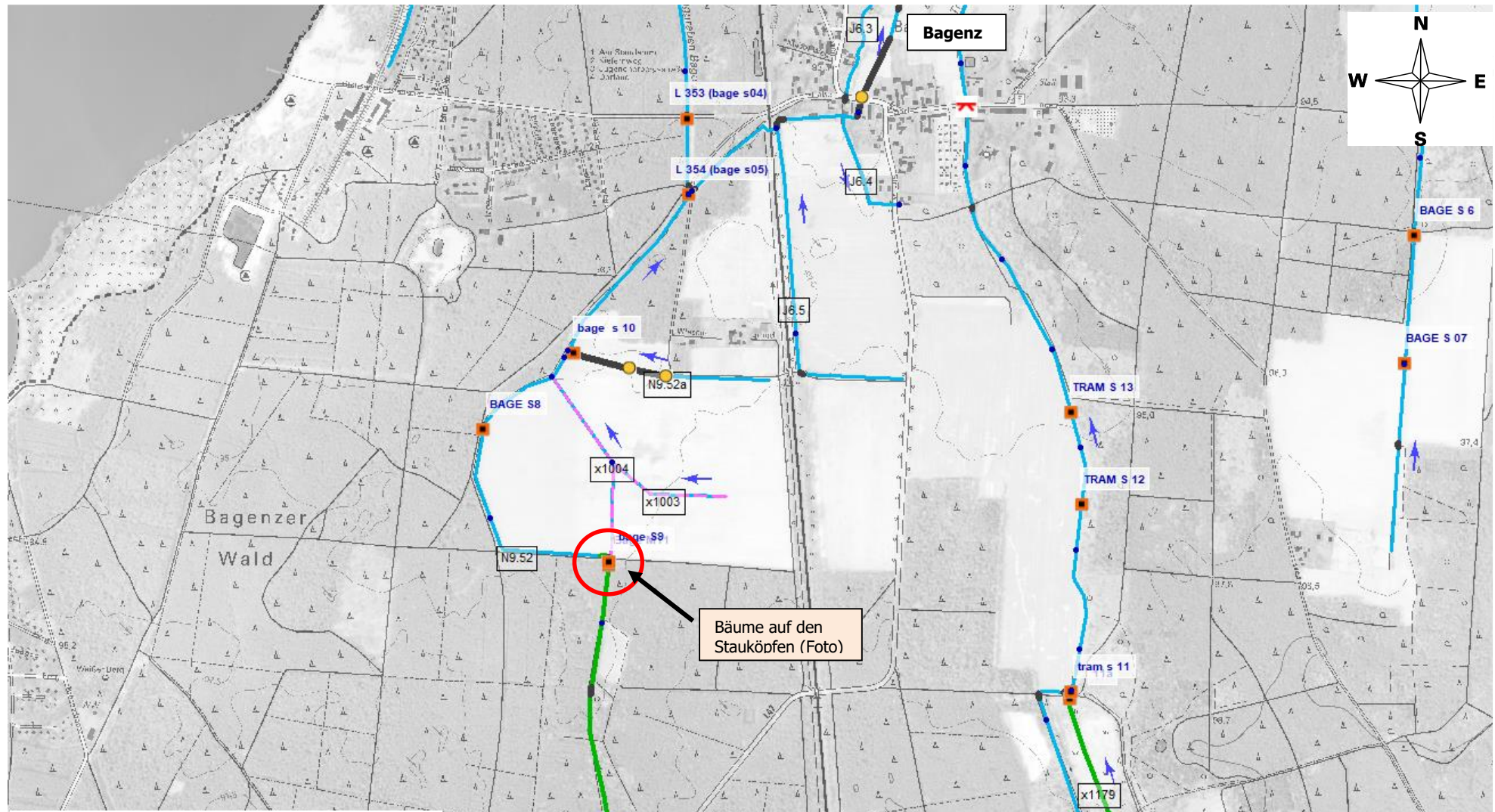
Gehölzplan Blatt N9.52 oberer Fanggraben Bagenz Bäume auf Bauwerken BAGE S 09 und Bage M11
